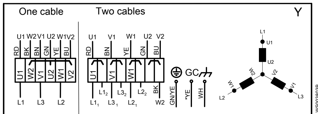
Рис. 15: Соединение звездой
