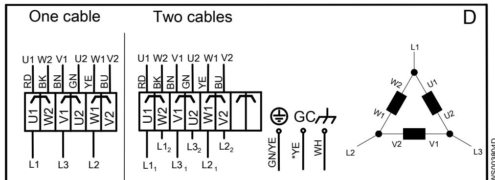
Рис. 16: Соединение треугольником
