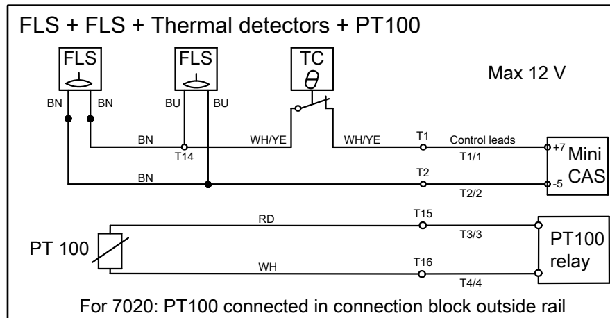
Рис. 25: 2 FLS + тепловые датчики + Pt100 (основной подшипник)
