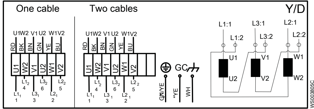
Рис. 17: «Звезда»/«Треугольник»
