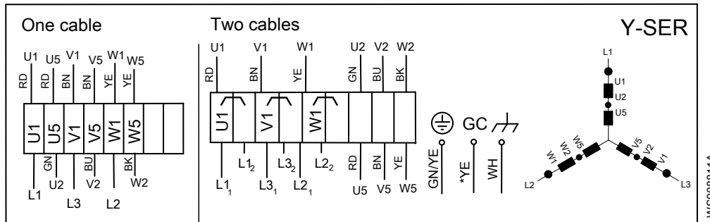
Рис. 19: Последовательное соединение звездой
