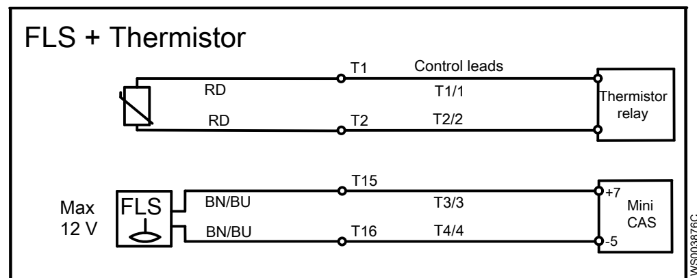
Рис. 26: 1 FLS + термистор
