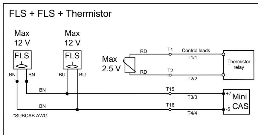
Рис. 27: 2 FLS + термистор
