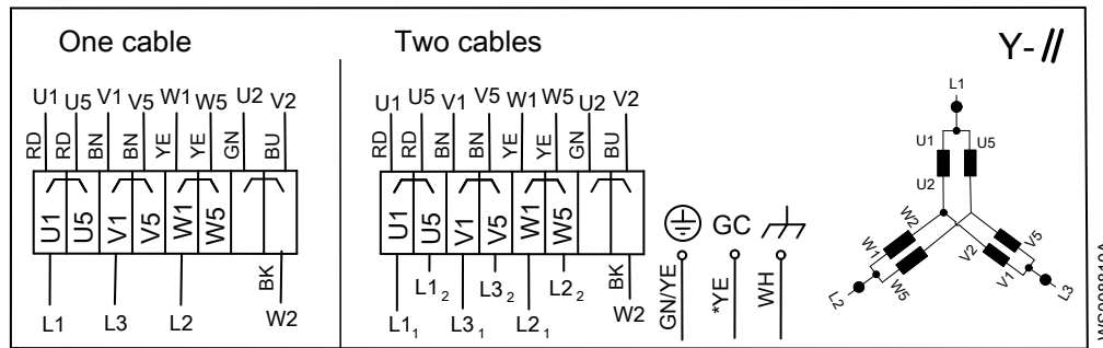
Рис. 18: Параллельное соединение звездой
