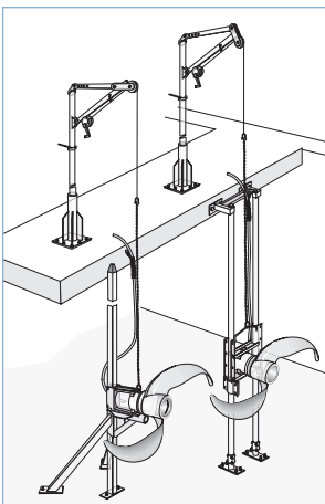
Установка с одной или двумя направляющими шинами Мешалки легко опускают и поднимают вдоль направляющих шин.
